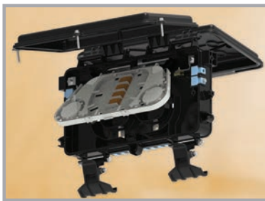
COYOTE® ATC
